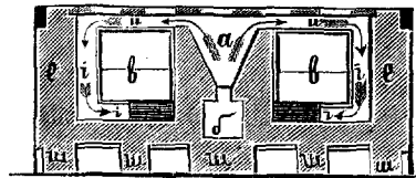
Вертикальный разрѣзь большого очага съ двумя шкафами и топливникомъ Свѣзева: а—топливникъ; б—зольникъ; в, в—духовые шкафы; и, и, и—шанцы; и, и—мѣсто для прохода дыма; е, е— боковыя стѣнки.
